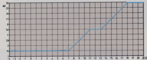
Blitzbelichtungscharakteristik
