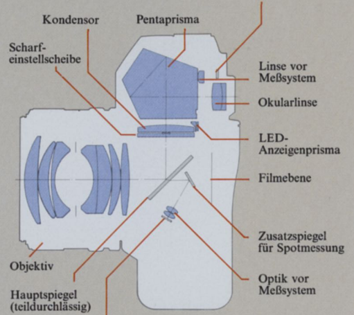
Meßzelle 2: Siliziumfotозelle für Spotmessung und für die Messung der Filmbereflächenreflexion
