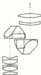
ZEISS Fernrohrvorsatz 8 x 30 B, Bildwinkel 6° DM 285.—
